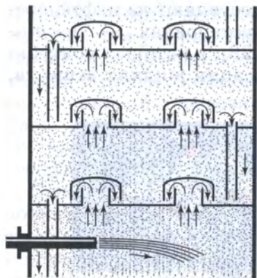
Рис. 29. Устройство тарелок ректификационной колонны
