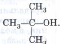
2-метилпропанол-2
