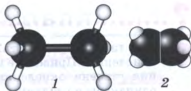
Рис. 7. Модели молекулы этана:
