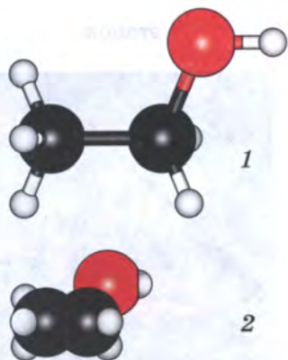
Рис. 37. Модель молекулы этанола: 1 — шаростержневая; 2 — масштабная
