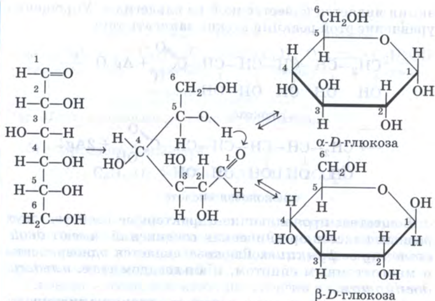
Рис. 66. Взаимопревращения циклической и линейной форм молекул глюкозы
