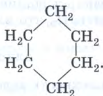
циклогексан
