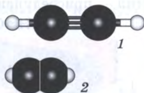
Рис. 21. Модели молекулы ацетилена: 1 — шаростержневая; 2 — масштабная
