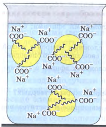
Рис. 62. Эмульгирование масла в воде в присутствии жира
