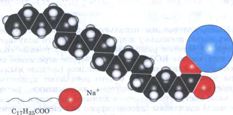
Рис. 61. Модель молекулы стеарата натрия в воде
