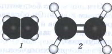
Рис. 14. Модели молекулы этилена: 1 — масштабная; 2 — шаростержневая
