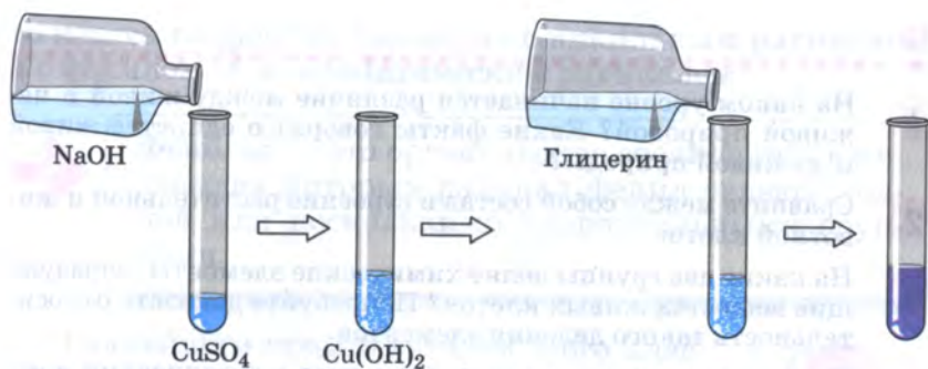
Рис. 41. Качественная реакция на многоатомные спирты
