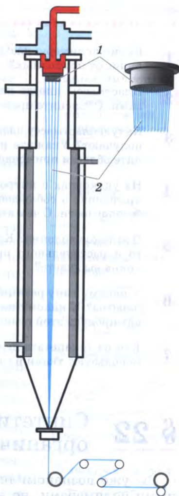
Рис. 83. Схема формирования волокон: 1 — фильера; 2 — пучок волокон
