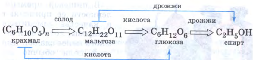
Рис. 67. Схема производства спирта из крахмала
