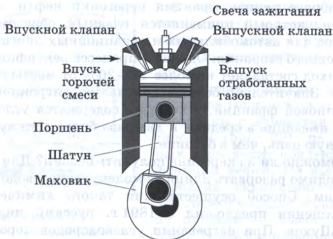
Рис. 30. Схема двигателя внутреннего сгорания
