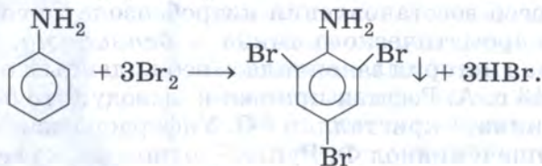
2,4,6-триброманилин
