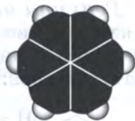
Рис. 25. Масштабная модель молекулы бензола
