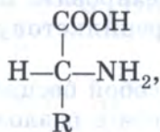
D -аминокислота
