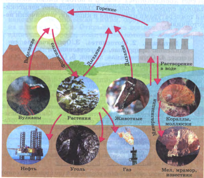
Рис. 5. Круговорот углерода в природе
