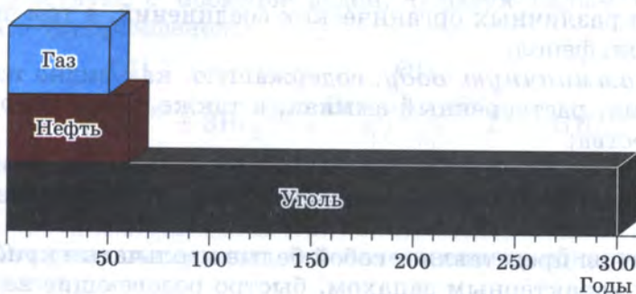
Рис. 43. Расчетное время потребления природных источников углеводородов
