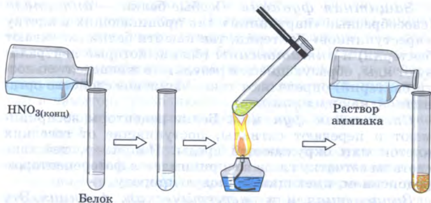
Рис. 78. Ксантопротеиновая реакция
