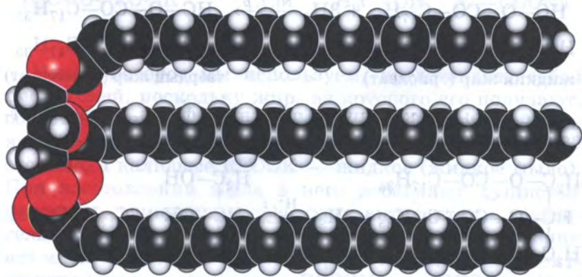
Рис. 60. Масштабная модель молекулы жира (тристеарата)
