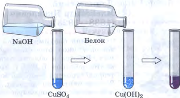
Рис. 77. Биуретовая реакция
