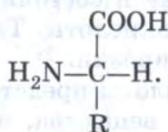
L -аминокислота
