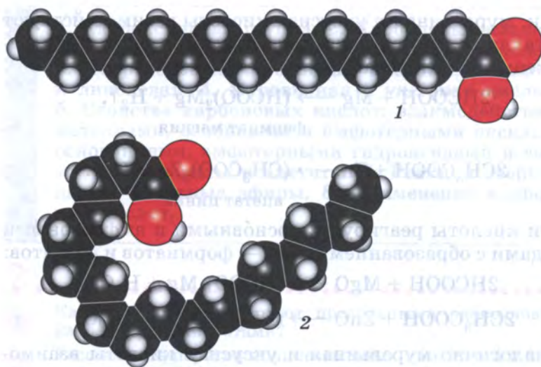
Рис. 56. Масштабные модели молекул:
