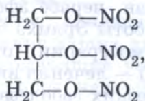
нитроглицерин
