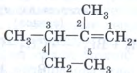
2,3-диметилпентен-1
