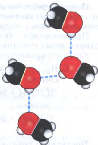
Рис. 32. Водородные связи между молекулами метанола
